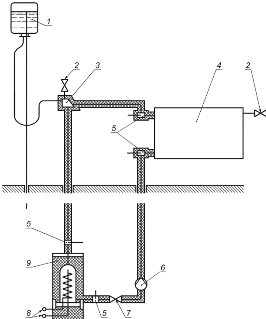
1 - расширительный бак; 2 - клапан воздухоотводчика; 3 - воздухоотделитель; 4 - испытуемый отопительный прибор; 5 - точки измерения температуры воды; 6 - насос; 7 - клапан; 8 - клеммы для присоединения к источнику напряжения; 9 - электрический котел
