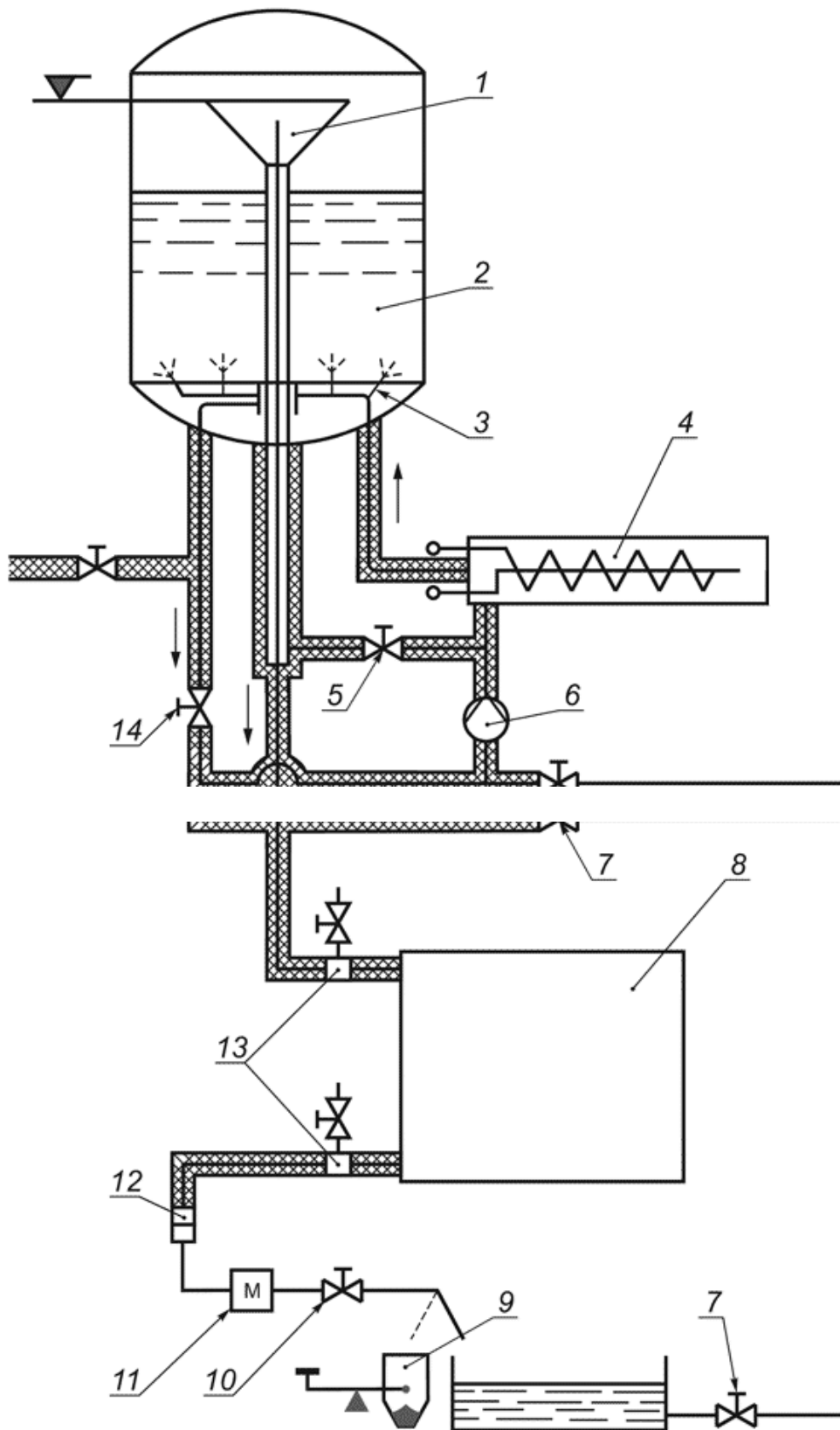
1 - перелив; 2 - бак постоянного уровня; 3 - смешивающее устройство; 4 - электрический котел; 5 - клапан; 6 - циркуляционный насос; 7 - клапан; 8 - испытуемый отопительный прибор; 9 - измерительный сосуд; 10 - клапан; 11 - теплообменник; 12 - фильтр; 13 - устройство для измерения температуры воды; 14 - клапан
