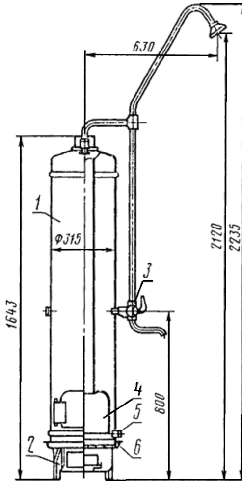
1 - водяной бак; 2 - подставка; 3 - смеситель; 4 - топка; 5 - сливной штуцер; 6 - наполнитель из смеси глины с асбестом
